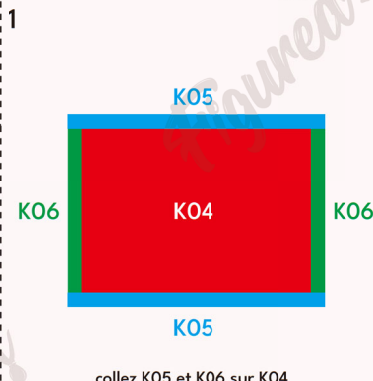
échelle:1:10 K06 plexiglas (transparent) 20*17.64*0.18 (2 pièces)
